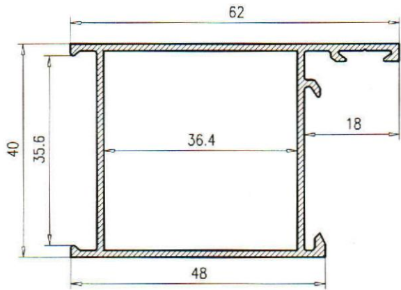
Marco 40*40 048
