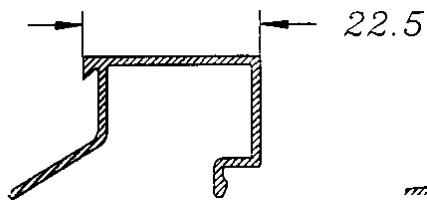
Junquillo 14 285
