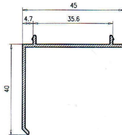
Premarco 40 040
