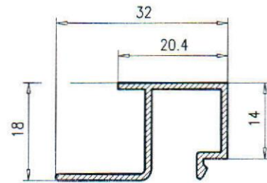
Junquillo 16 286
