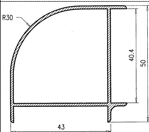
Esquinero 40
