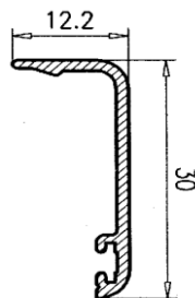
Premarco Cajón 30 039
