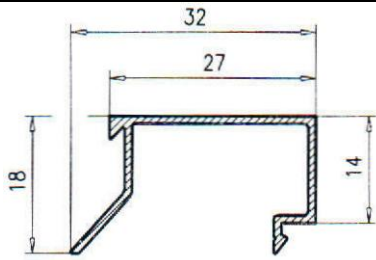
Junquillo Normal 199
