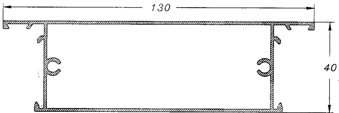
Pilastra Zócalo 416
