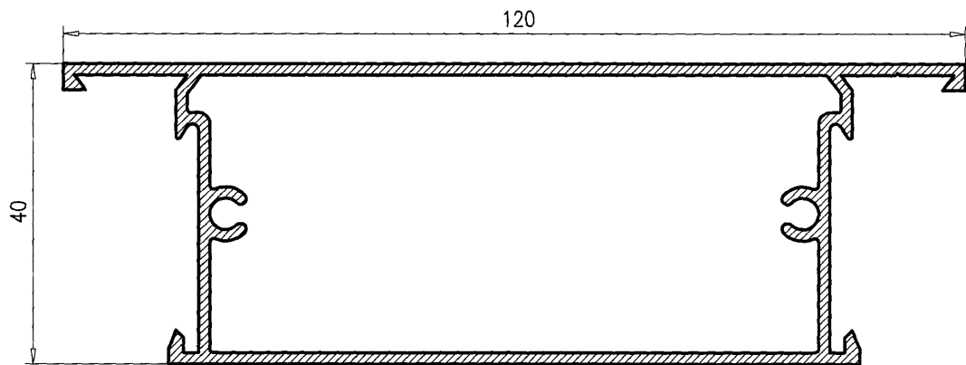
Pilastra Zócalo 120 415
