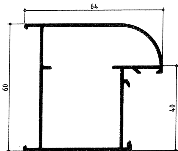
Marco Escaparate 050
