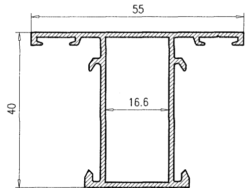
Pilastra 40*20 063
