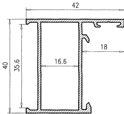
Marco 40*20 562
