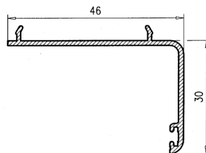
Premarco 30 041
