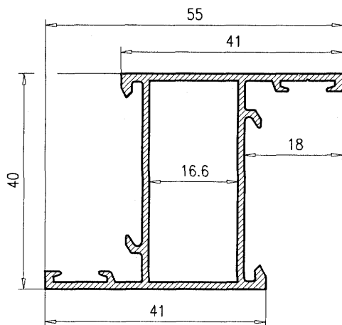
Hoja 40*20 663
