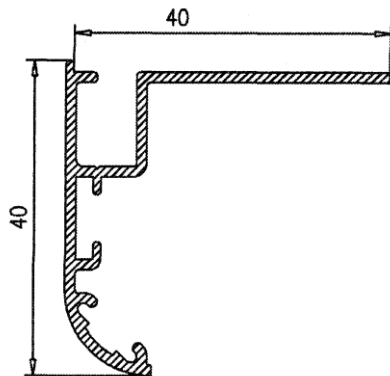
Premarco 40*40 031
