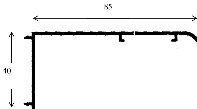
Premarco Cajón 30 039
