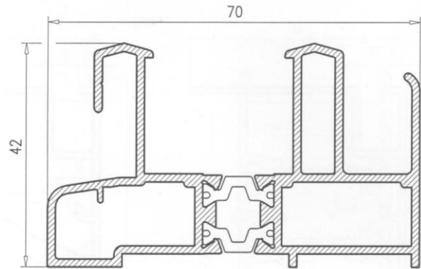
Marco de 70 Perimetral RPT 17200
