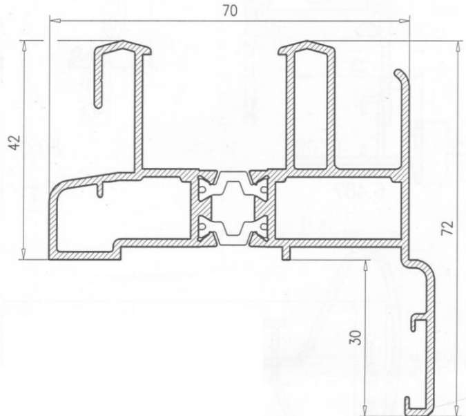
Marco de 70 Perim. con premarco RPT 17260
