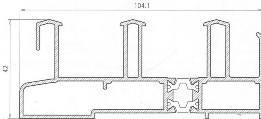
Marco 3 carriles RPT 17201
