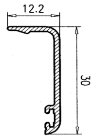
Tapa Cajón 039
