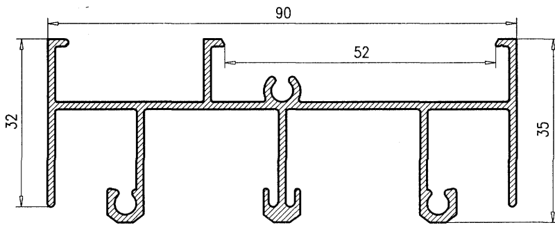
Marco Superior 3 carriles 702
