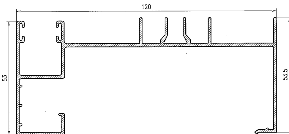
Marco Lateral con Guía de 120 izquierda
