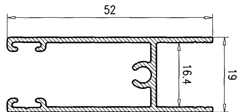
Hoja Rueda c/16 7018
