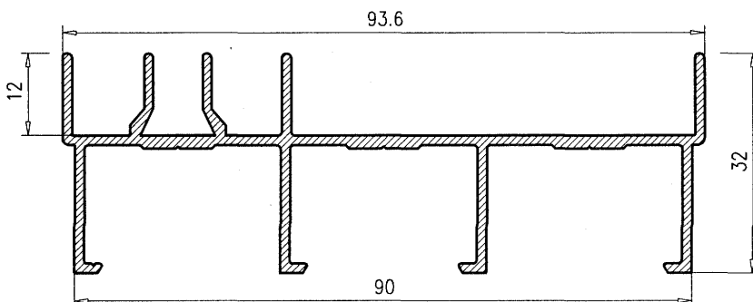
Marco Lateral 3 carriles 703
