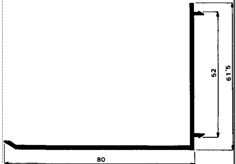
Premarco 80 060
