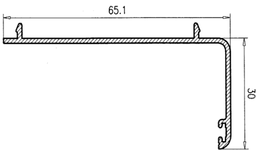
Rotula 60 7000
