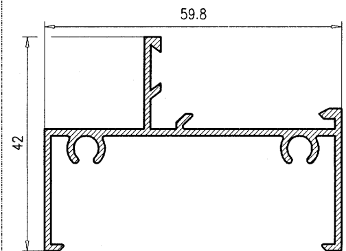
M. Fijo Hembra 481
