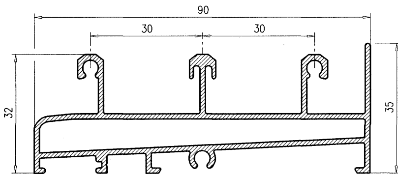
Marco Inferior 3 carriles 701
