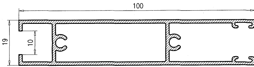
Zócalo Normal 7022
