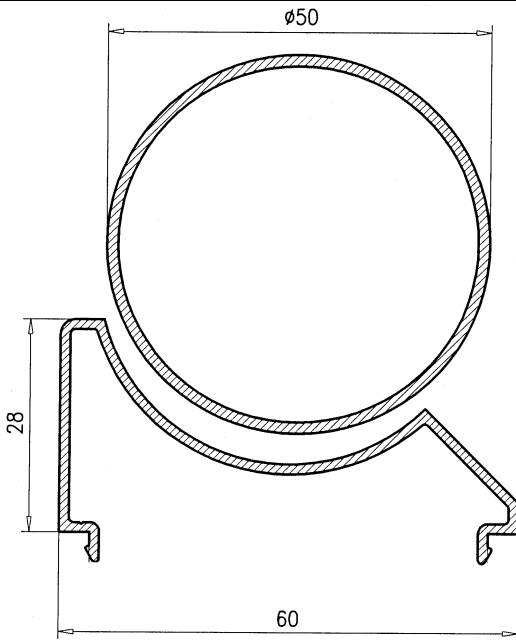
Rotula 60 7000
