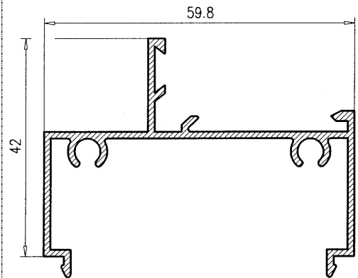
M. Fijo Macho 484
