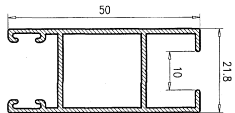
Hoja Lateral 50 7025
