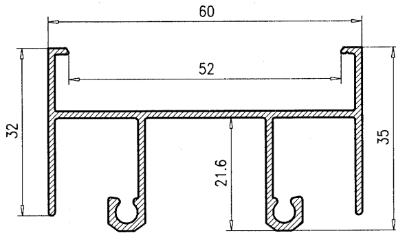
Marco Superior 7102
