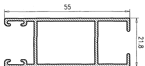
Hoja Lateral 55 7026
