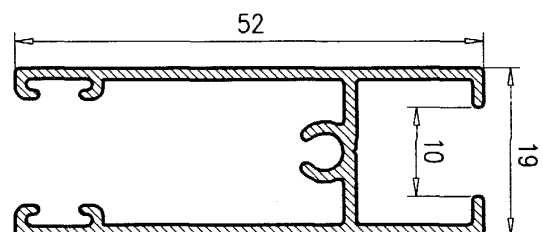
Hoja Rueda 7027
