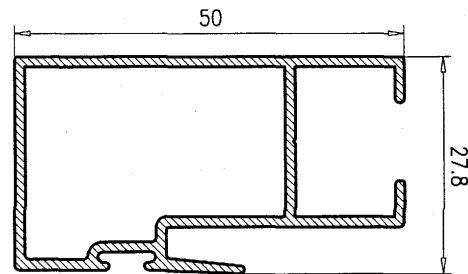
Hoja Central 50 7023
