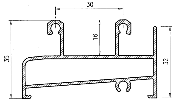
Marco Inferior 7101
