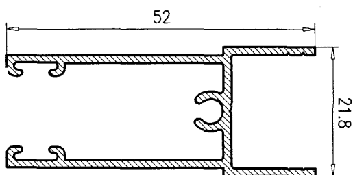
Hoja Rueda Climalit 7010
