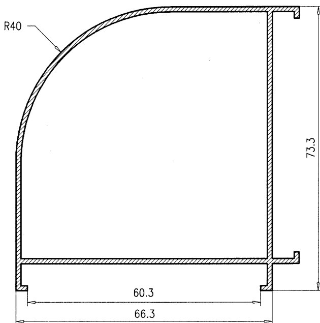
Esquinero 60 049
