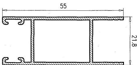
Hoja Lateral Climalit 55 7012
