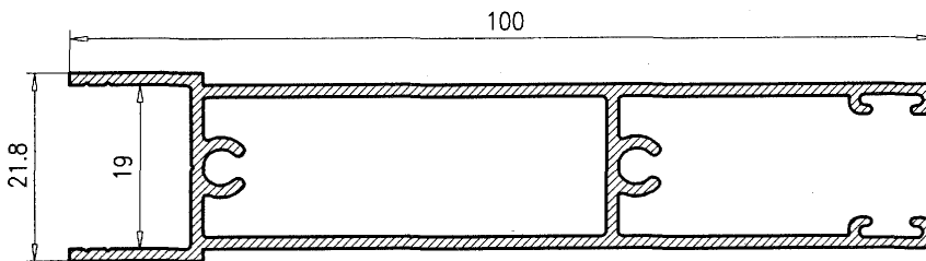
Zócalo Climalit 7020
