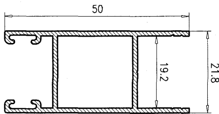
H. Lateral Climalit 50 7014
