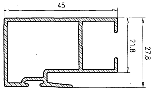
Hoja Central 45 7024
