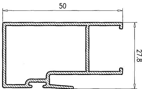
Hoja Central 50 c/16 7017
