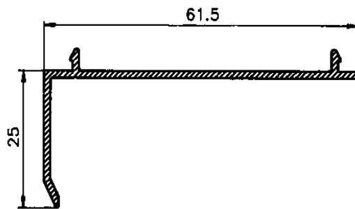
Premarco 25 025
