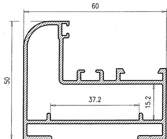
Marco Escaparate 121283
