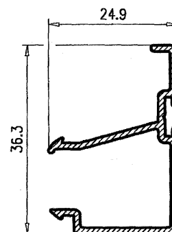
Junquillo Vaivén 122714
