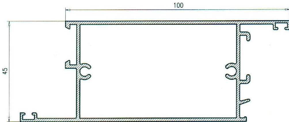
Hoja Zócalo 123477
