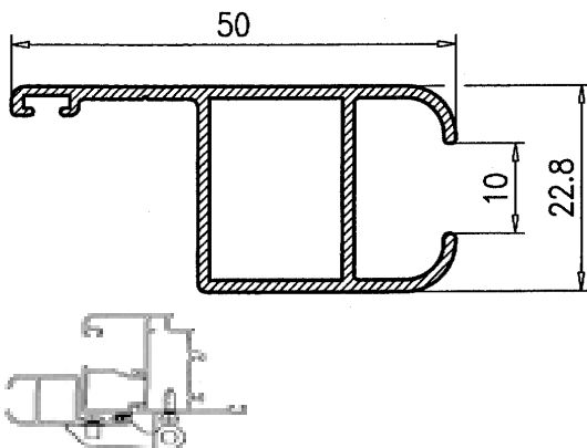
Contraventana 122080
