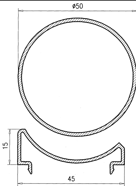
Rotula Abatible 45 122722
