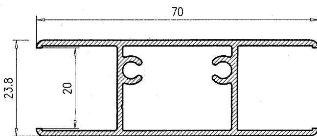
Parteluz Climalit 116217
