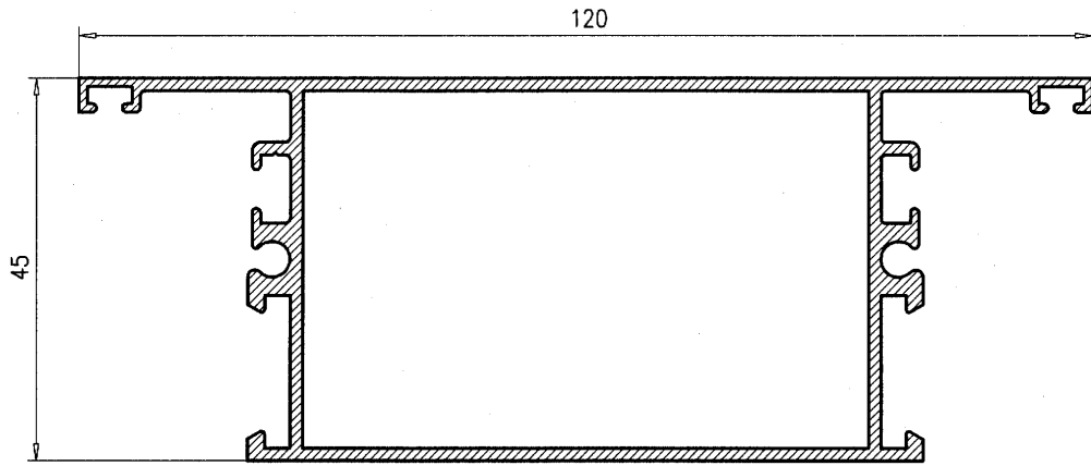
Pilastra Zócalo 123478
