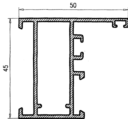
Marco Ventana 122280
