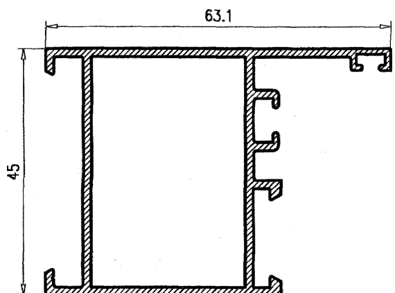
Marco Puerta 123280
