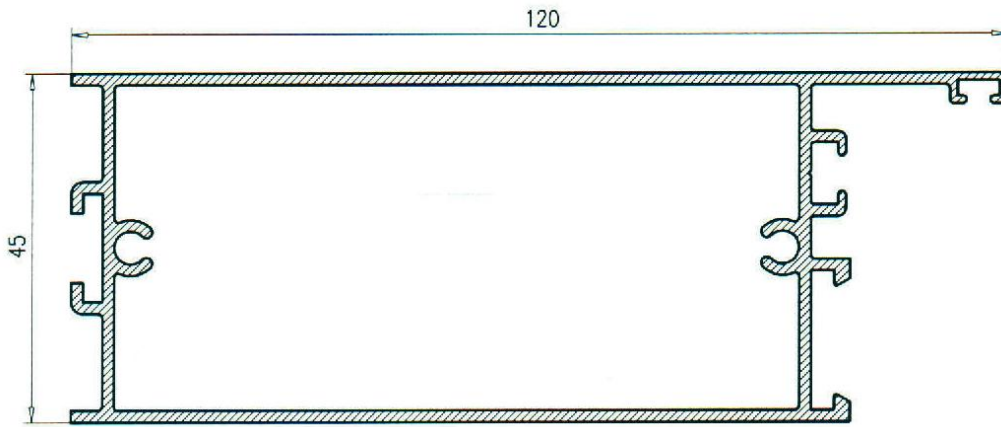
Marco Zócalo 123476
