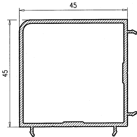
Esquinero 90 7058
