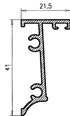
Marco Inferior 123486
