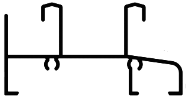
Marco Inferior sin cámara 124231
