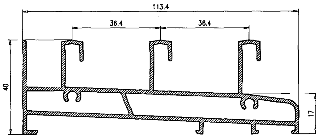
Marco Inferior 3 carriles 911
