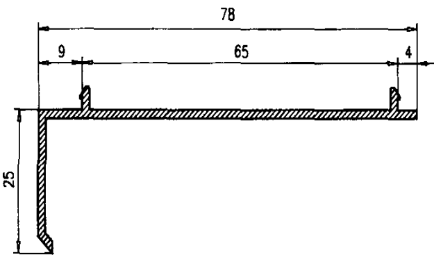
Unió Corredera 215
