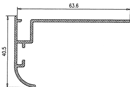
Solape 40 Cataluña 032
