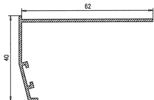
Solape 40 Recto 033
