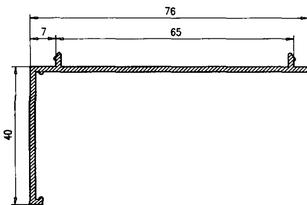
Premarco 40 045
