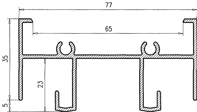
Marco Superior 124220
