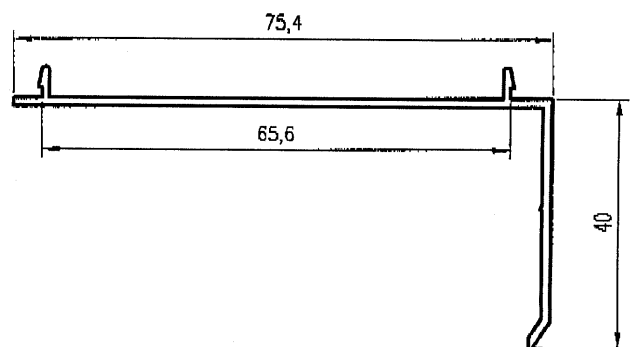
Premarco 30 036
