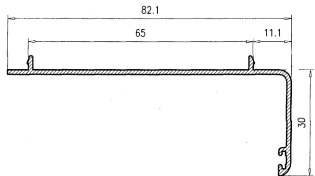
Unió 80-40 216
