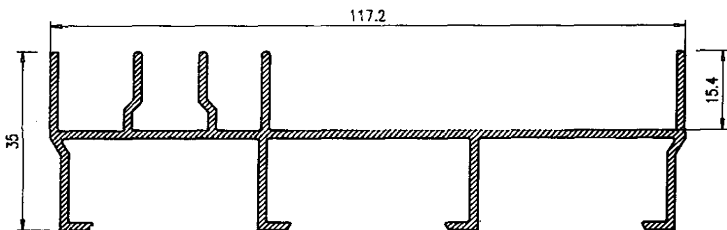
Marco Inferior 3 carriles 911
