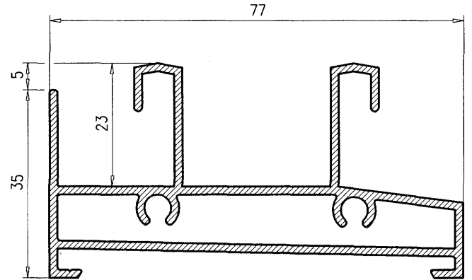
Marco Inferior 124230
