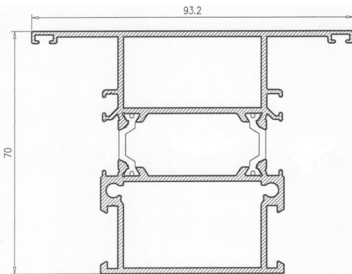
Pilastra Puerta 2670580
