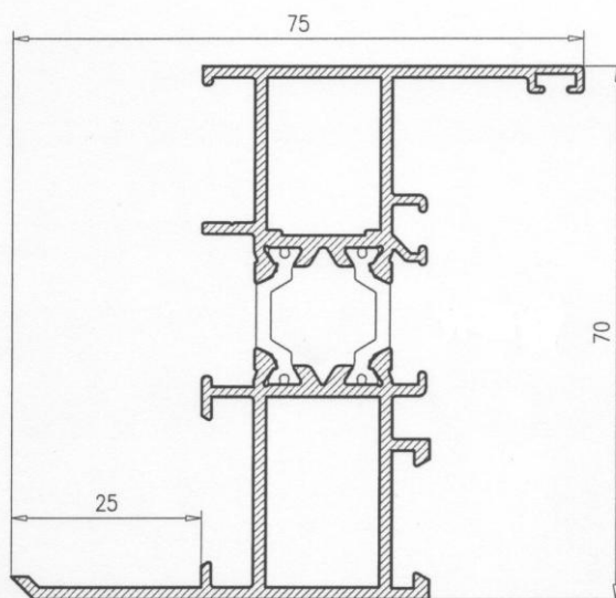
Marco Ventana 2570280
