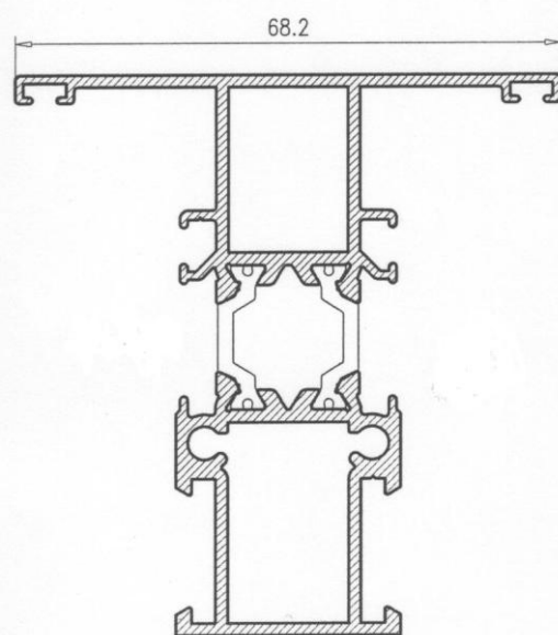
Pilastra Ventana 2570580
