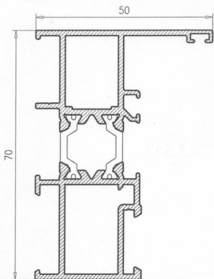
Marco Ventana 2570280
