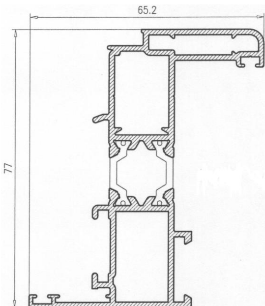
Hoja Ventana 2570380
