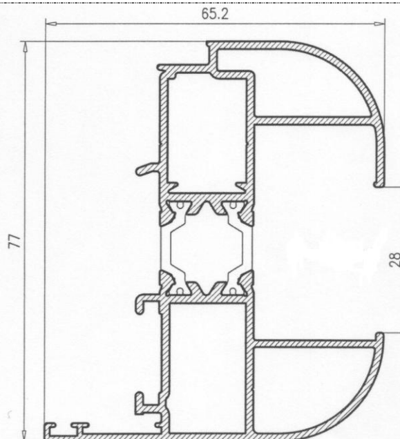
Hoja Ventana 2570380
