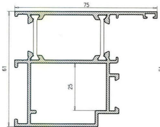
Marco Puerta Enrasado 37281
