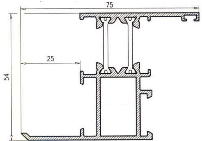
Marco Ventana. Solape 36282
