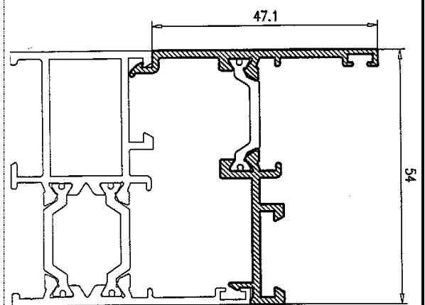
Inversor de marco 36384
