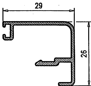
Junquillo Base 29 hueco 21.5 36262
