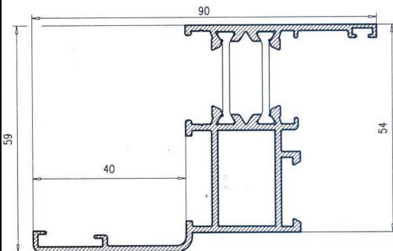
Marco Ventana Solape 36281
