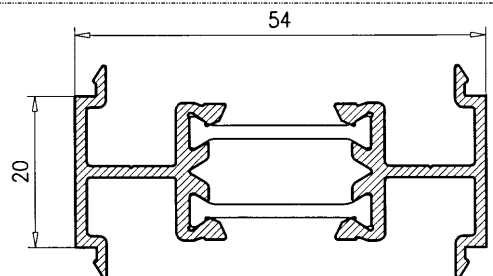
Marco Ventana c/solape 36283
