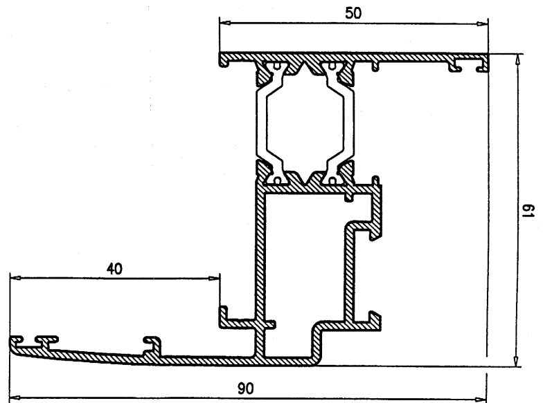
Marco Ventana c/solape 36283
