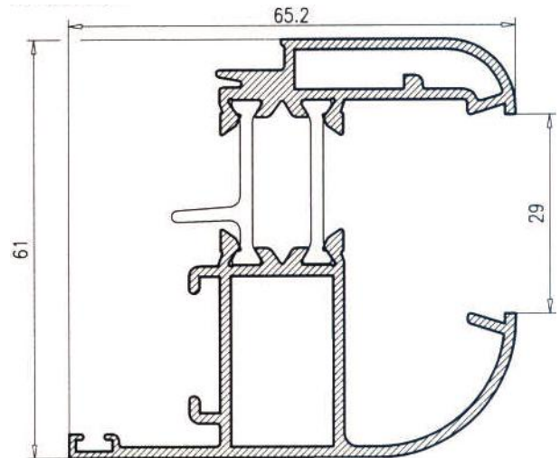
Hoja Ventana s/junquillo 36382
