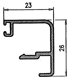
Marco Ventana c/solape 36283
