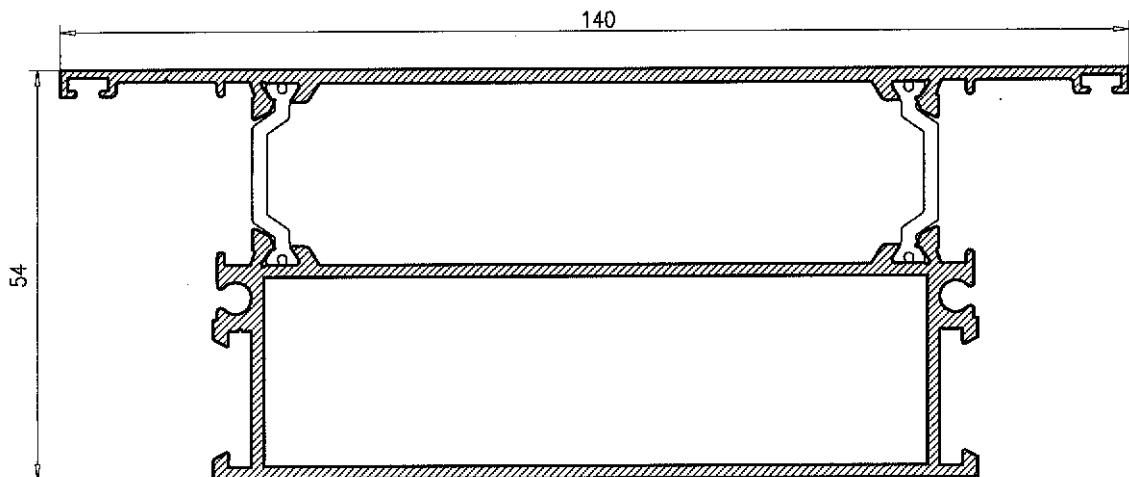
Pilastra Zócalo 37476
