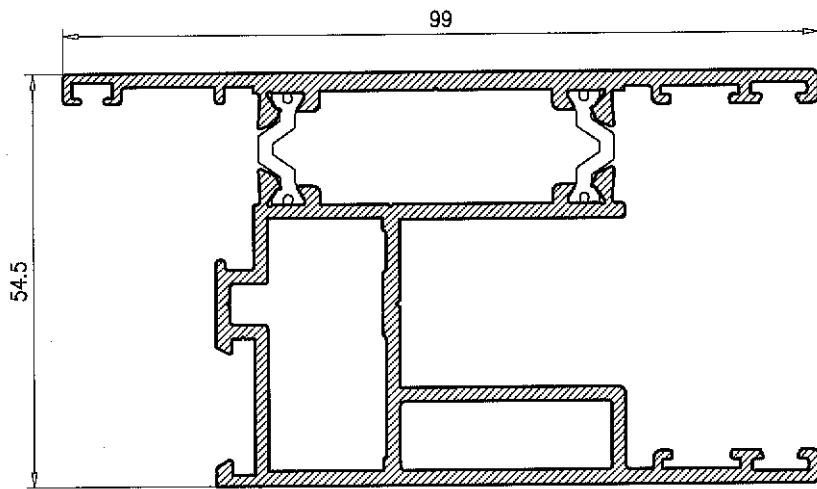
Hoja Perimetral 63
