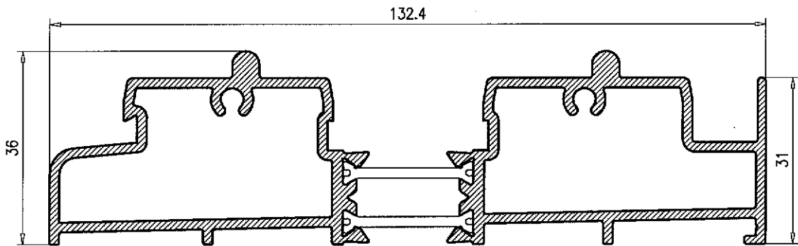
Marco Inferior 61
