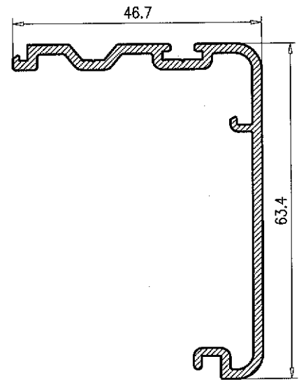
Cruce Central 66
