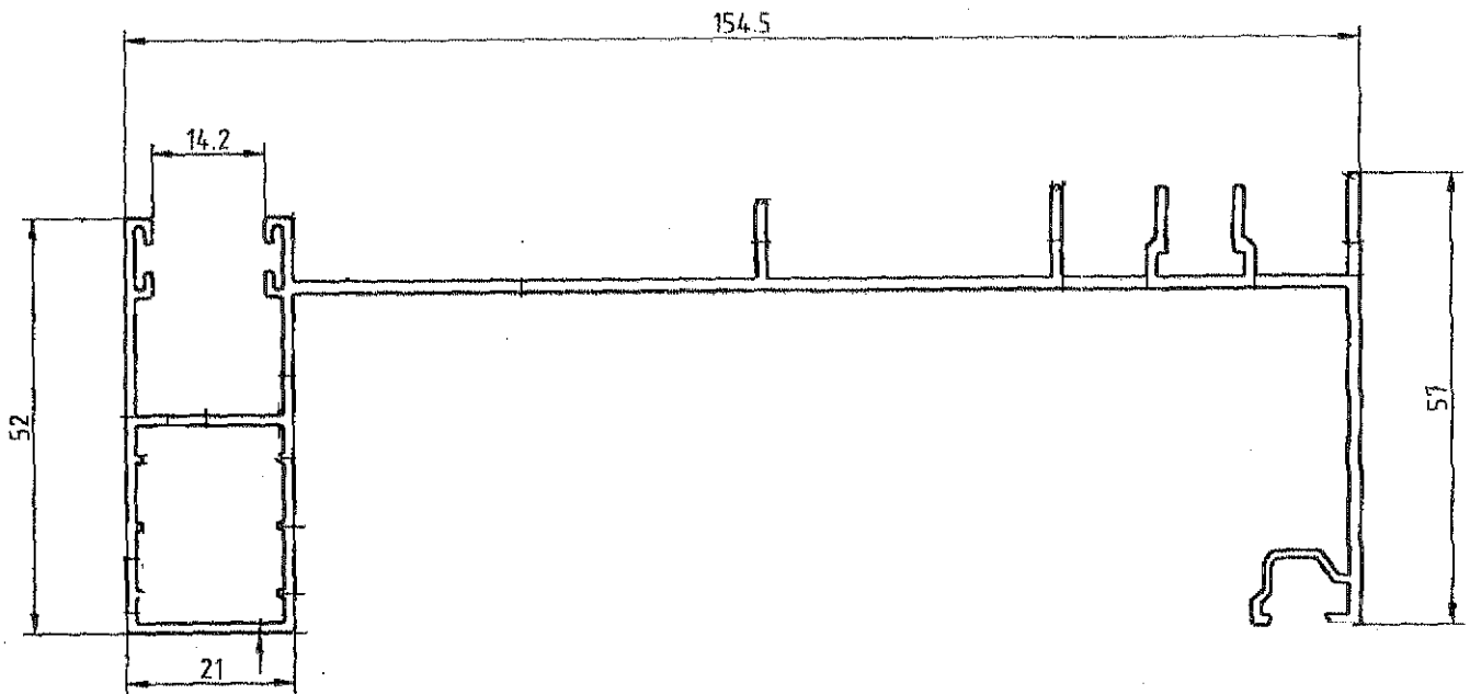
Marco Lateral Compacto Derecho 154.5 7206
