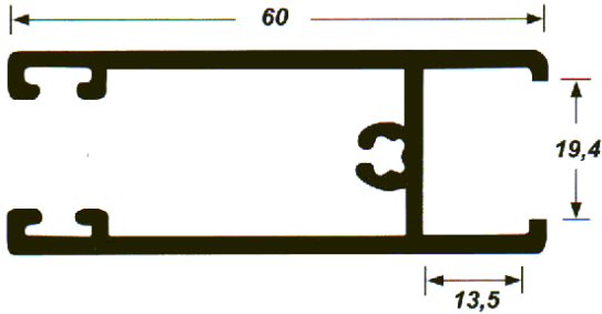
Hoja Rueda Climalit 7210
