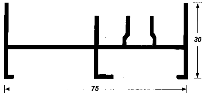
Marco Lateral Nuevo 7227
