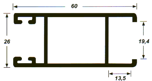
Hoja Lateral Climalit 7214
