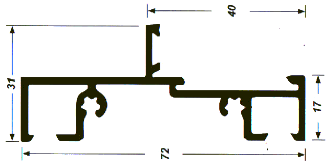
Marco Fijo Hembra 7281
