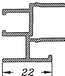
Cierre 4 hojas 808
