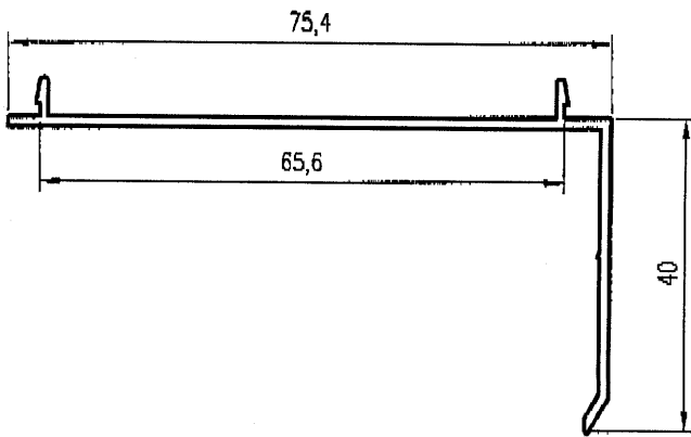
Premarco 40 biselado 046
