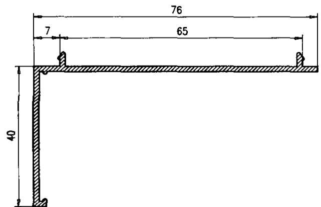
Premarco 40 045
