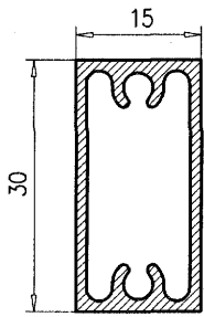
Rect. 30*15 aut. 472
