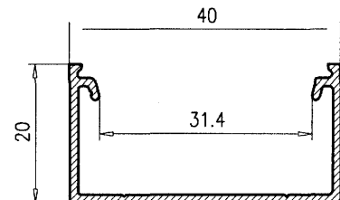
Forma U 20 801
