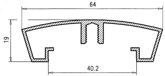
Pasamano autorroscado 127
