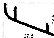
Tapa anclaje 796
