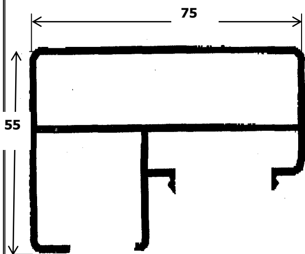
Anclaje Cristal 797
