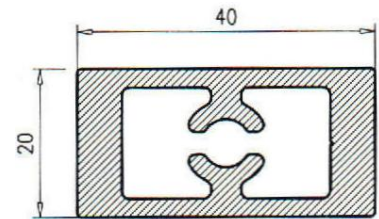
R. 40*20 aut. 7442
