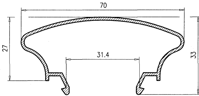
Pasamano Barandilla 321
