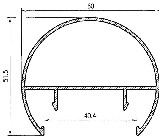
Pasamano Barandilla 321
