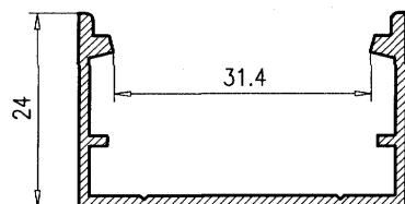
Forma U 25 799
