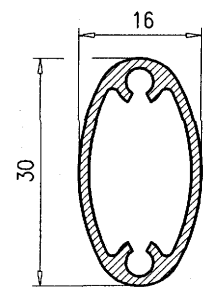
Ovalado aut. 830
