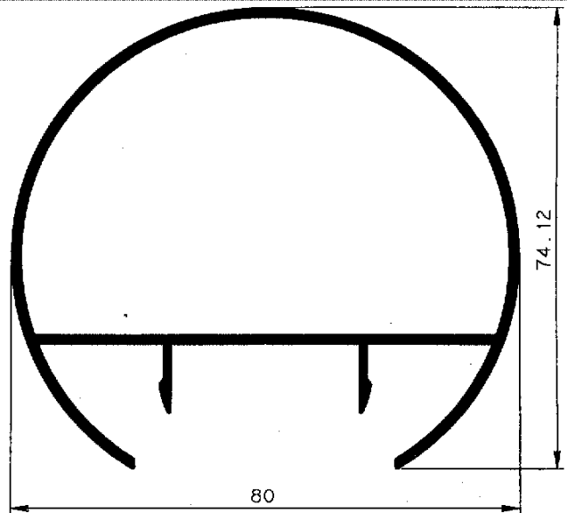
Pasamano Redondo 80 323
