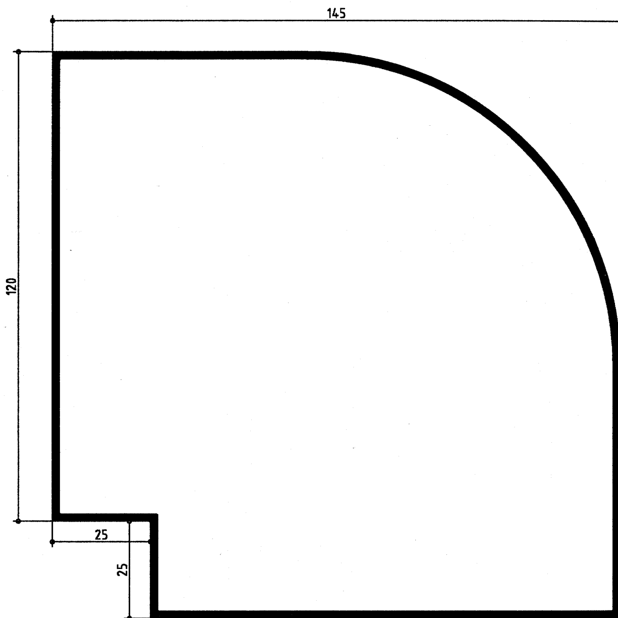
Esquinero Compacto 145
