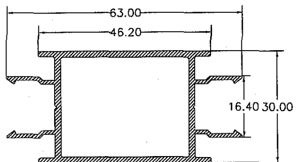
Mampara doble 508
