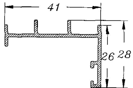
Perfil Cerco 504
