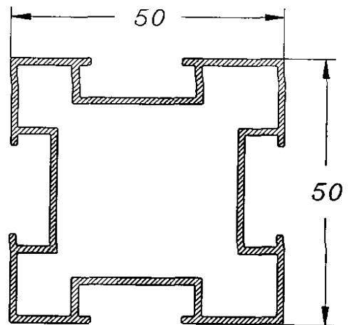
Perfil 4 Salidas 502
