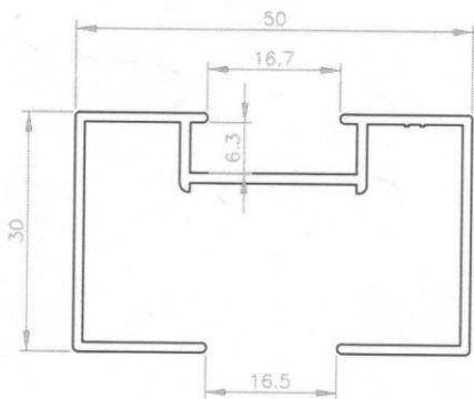
Perfil 1 Salida 03112
