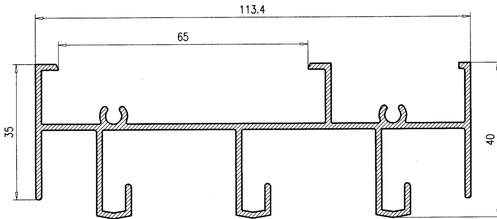
Marco superior tres carriles 912
