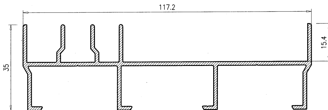
Marco lateral tres carriles 913
