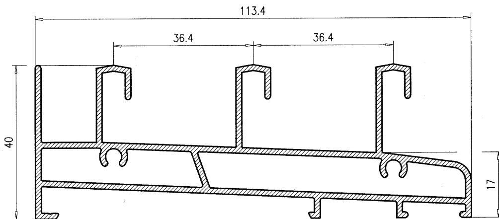
Marco inferior tres carriles 911
