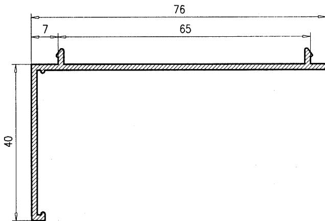
Premarco de 40 045
