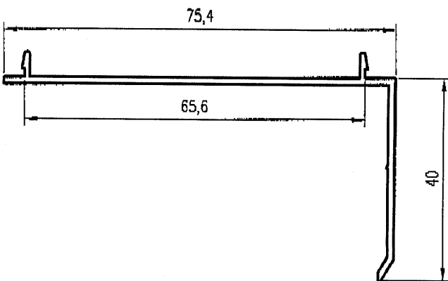
Premarco 40 biselado 046
