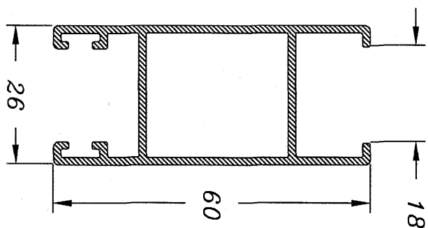
Hoja Lateral Climalit 98
