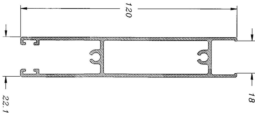
Zócalo Climalit 903
