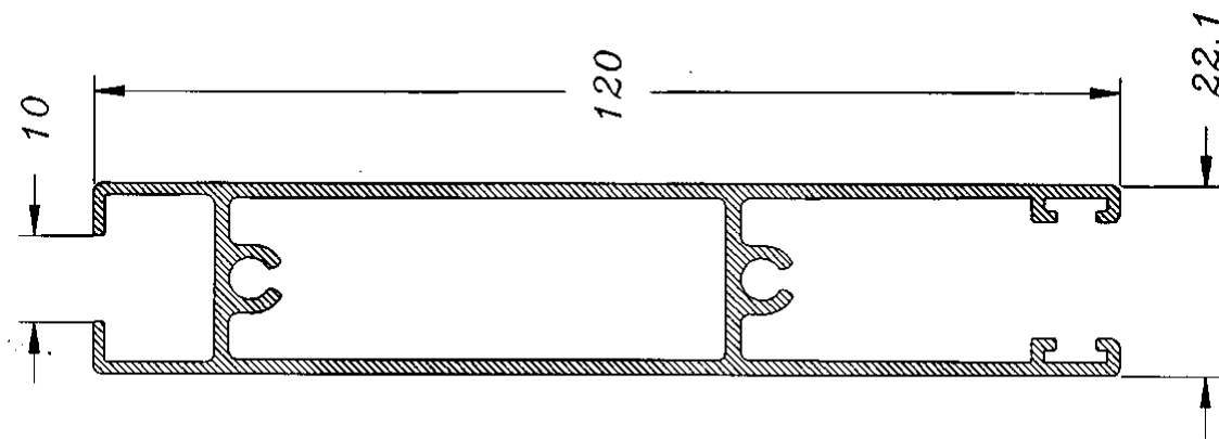
Zócalo Normal 97
