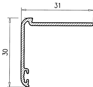
Premarco 30 030
