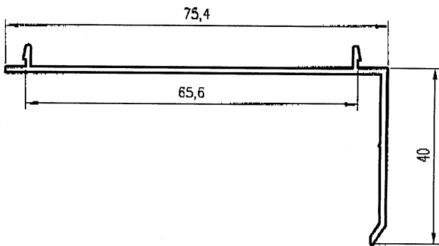
Premarco 40 biselado 046
