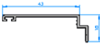
Premarco 43 atornillado 72702
