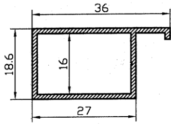
Premarco obra 36 506
