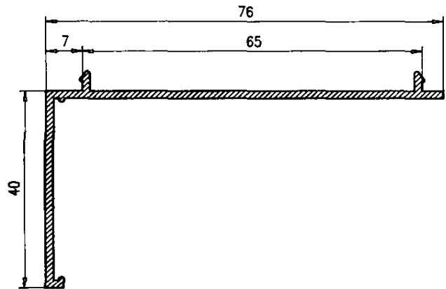
Premarco 60 atornillado 72703
