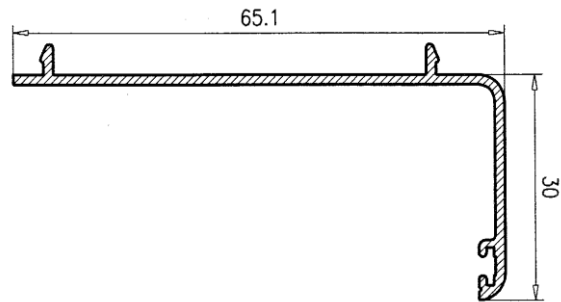
Premarco 30 042
