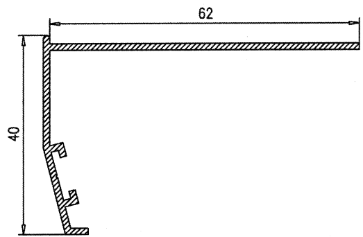
Solape 40 recto 033
