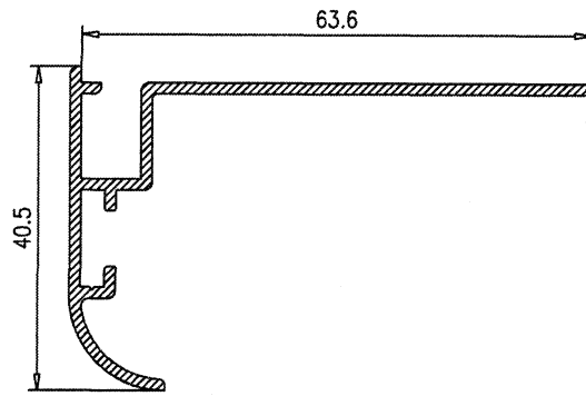
Solape 40 Cataluña 032
