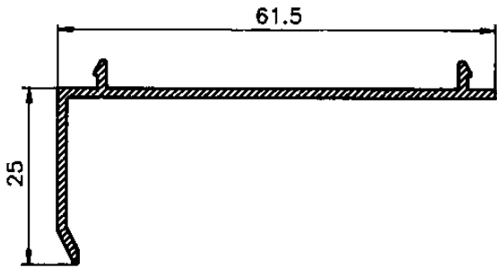
Premarco 25 025
