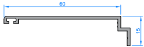
Premarco 60 atornillado 72703
