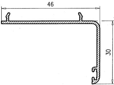
Premarco 30 041
