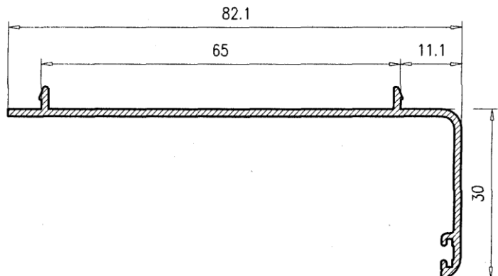
Premarco 30 036
