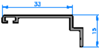
Premarco 33 atornillado 72701
