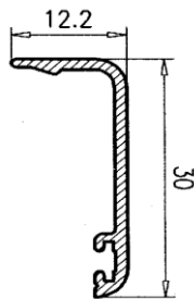
Tapa Cajón 039
