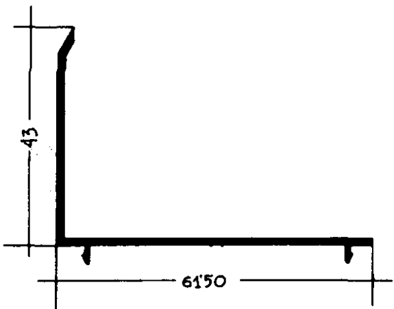
Premarco 43 043
