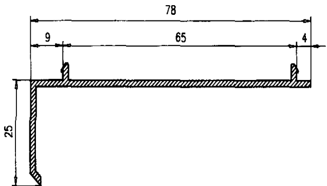
Premarco 25 922
