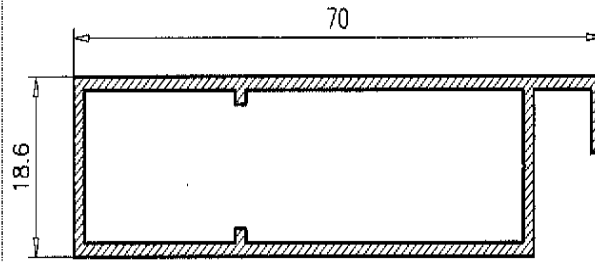
Premarco obra 36 506
